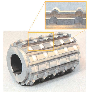
多山スプラインカッタ
