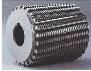
多山ラックカッタ
