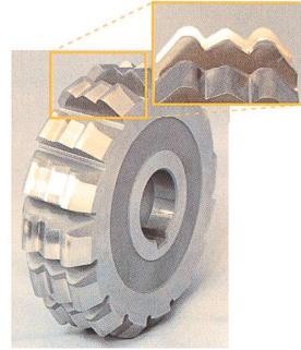
フォームドカッタ
