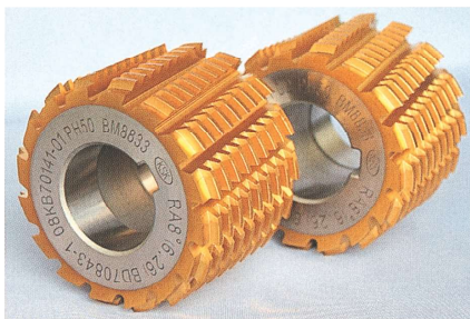
高精度組み合わせカッタ
